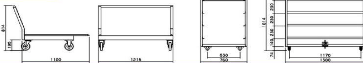
運搬・処理台車仕様例
